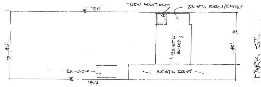
SITE PLAN SCALE: 1" = 20'
